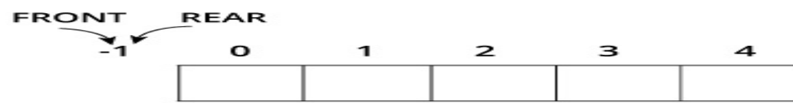
Empty Queue
